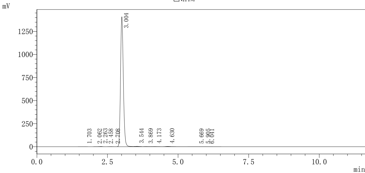
色谱图
